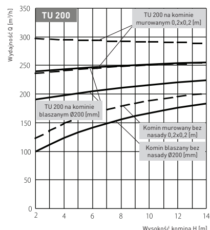
Wykres wydajności obrotowej nasady kominowej TURBOWENT Ø200 dla kominu blaszanego i murowanego, dla dwóch prędkości wiatru 3 i 4 [m/s].
