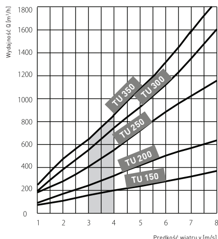
Wykres wydajności obrotowych nasad kominowych TURBOWENT w zależności od prędkości wiejącego wiatru bez uwzględnienia wysokości kominu. (*1[m/s]=3,6[km/h]).
