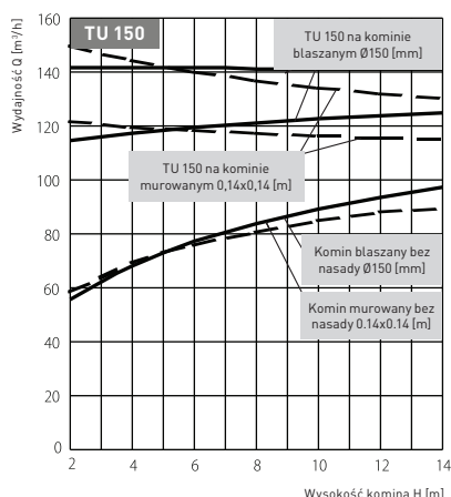
Wykres wydajności obrotowej nasady kominowej TURBOWENT Ø150 dla kominu blaszanego i murowanego, dla dwóch prędkości wiatru 3 i 4 [m/s].
