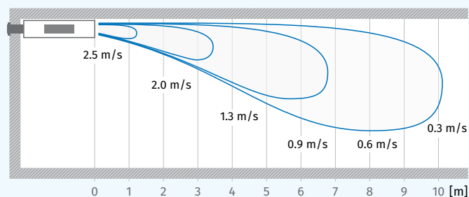
Zakres rozchodzenia się strumienia powietrza dla CIVIC EC DB 500
