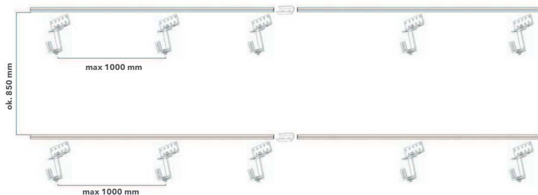
Rys. 2 Rozmieszczenie szyn montażowych wraz z uchwytem regulowanym. Maksymalna długość szyny za mocowanie bez podparcia < 250mm
