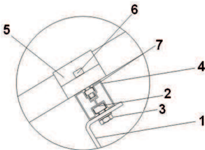
Rys. 4 Mocowanie modułów do szyny montażowej
