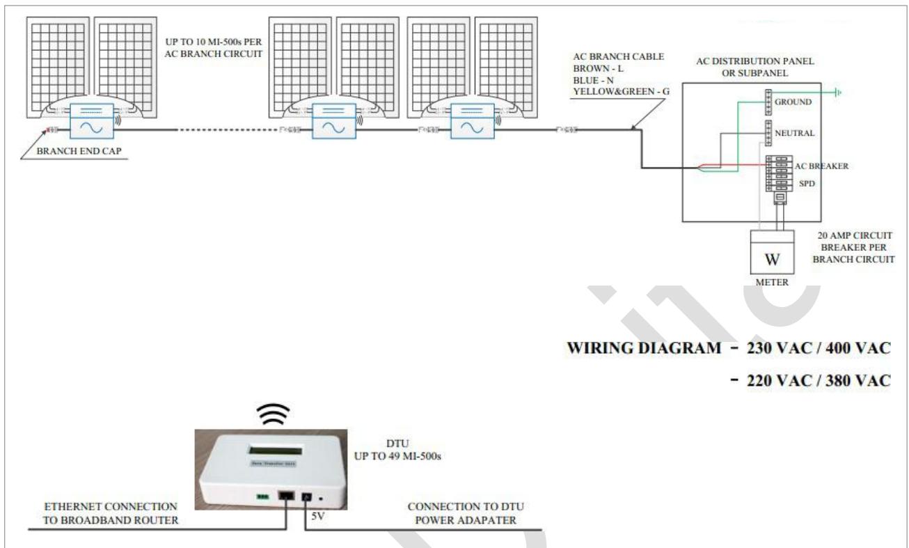
Rys. 2 Schemat połączeń jednofazowych
