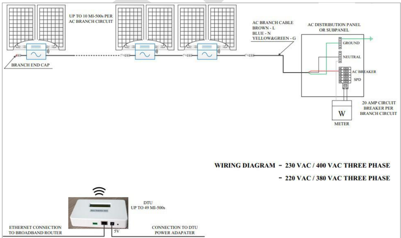
Rys. 3 Schemat połączeń trójfazowych
