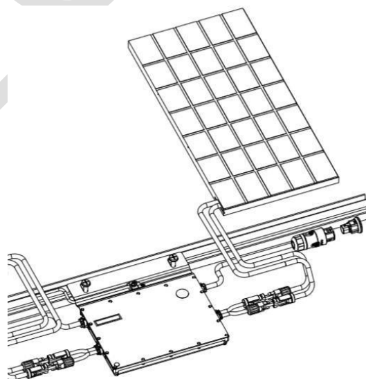
Rys.1 Pozycja montażowa mikroinwertera
